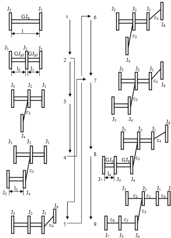
Динамические модели привода исполнительных механизмов швейных машин базы 97 кл
