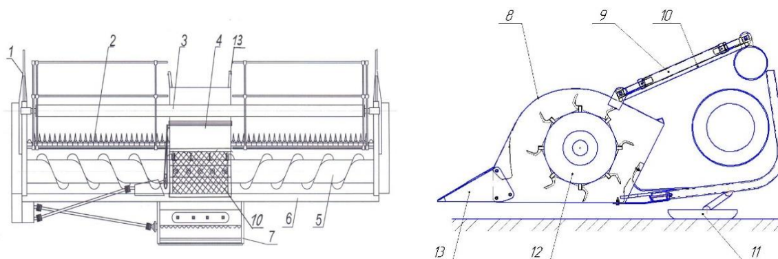
Рис. 2. Схема хедера с очесывающим адаптером для формирования стерневых кулис: 1 – делители растительной массы; 2 – режущий аппарат; 3 – мотовило; 4 – очесывающая приставка; 5 – шнек; 6 – рама хедера; 7 – проставка; 8 – кожух; 9 – регулируемые тяги; 10 – сетка; 11 – башмаки; 12 – очесывающий барабан; 13 – делители
