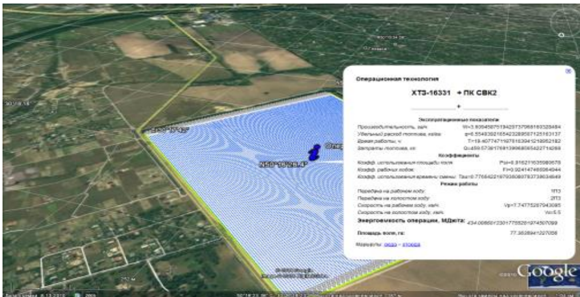
Рис. 4. Вид проведенных компьютерных экспериментов на примере почвообрабатывающе-посевного комплекса со второй схемой компоновки с помощью разработанной автоматизированной системы моделирования
