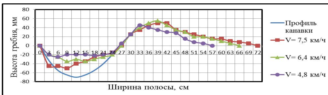
Рис. 2. Профиль следа и профиль канавки от кольца диаметром 700 мм установленного под углом атаки 28 град.
