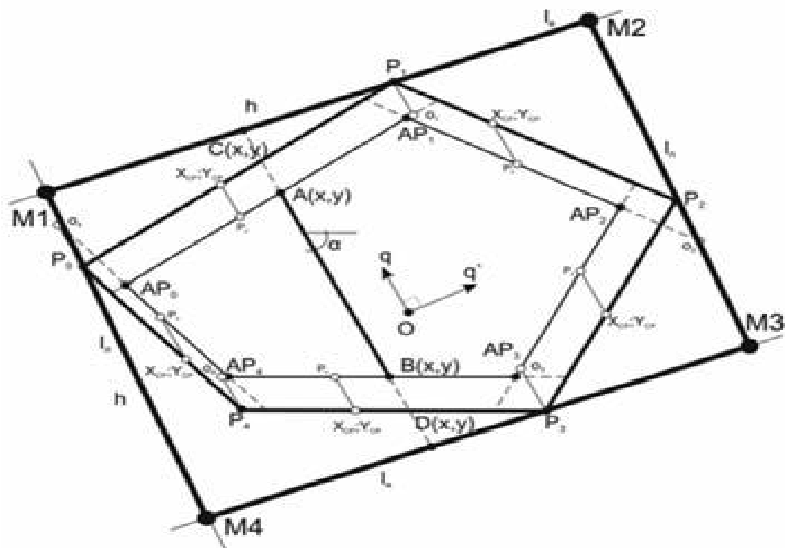
Рис. 2. Построение активной зоны и рабочего хода
