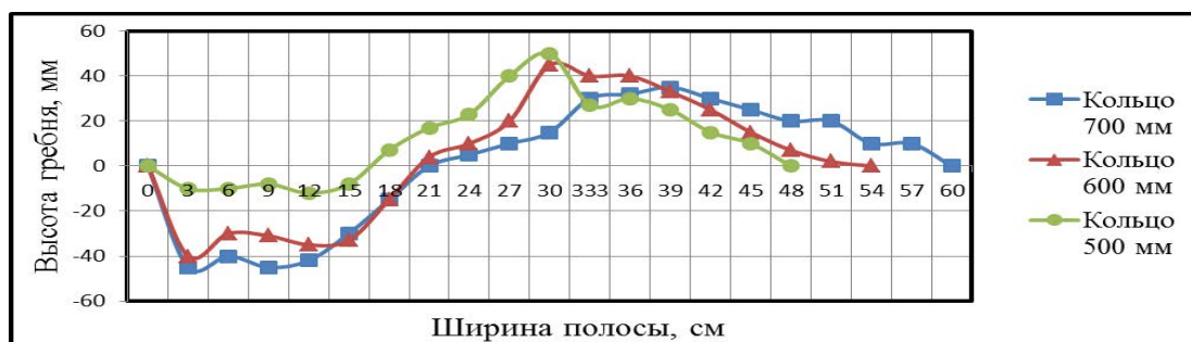
Рис. 3. Профиль следа от колец диаметром 500, 600 и 700 мм, установленных под углом атаки 24 град. и движущихся со скоростью 7 км/ч
